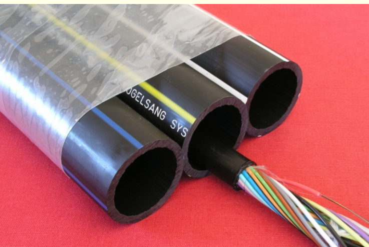
Mehrfachrohr des Standards „dreifach DN50“
